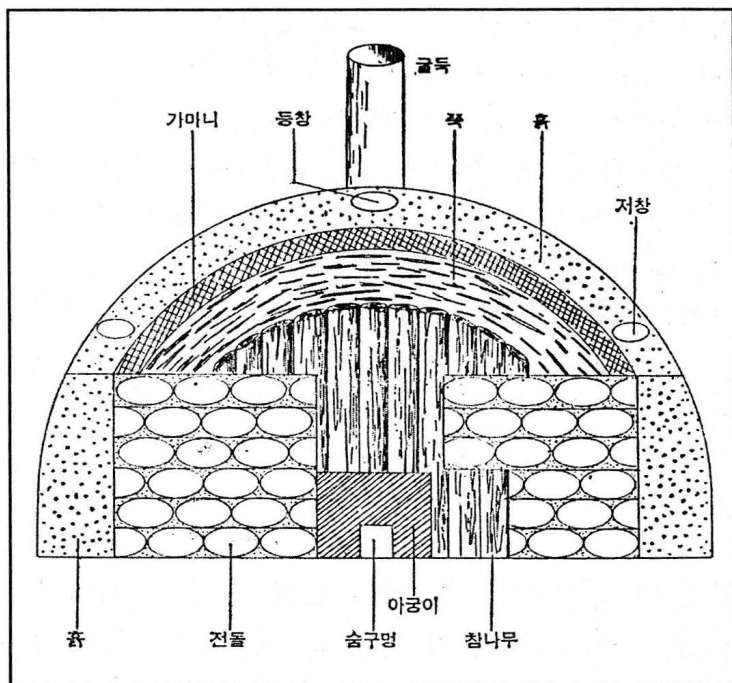
- 숯가마의 구조 -
