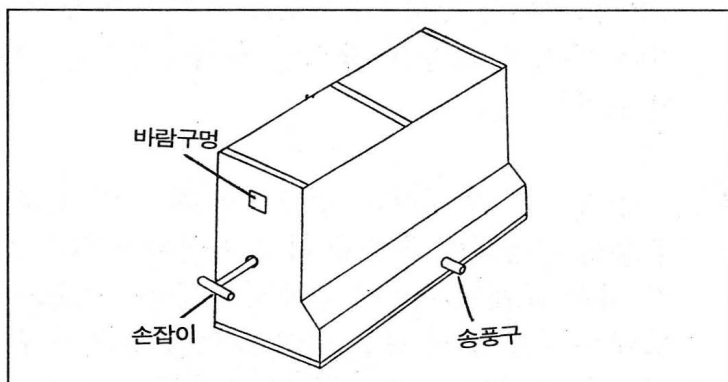
— 나무상자 풀무 —
